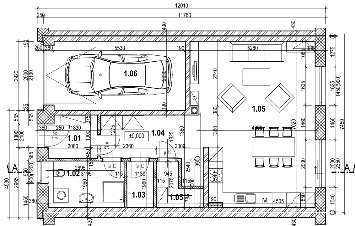
1. NADZEMNÍ PODLAŽÍ
