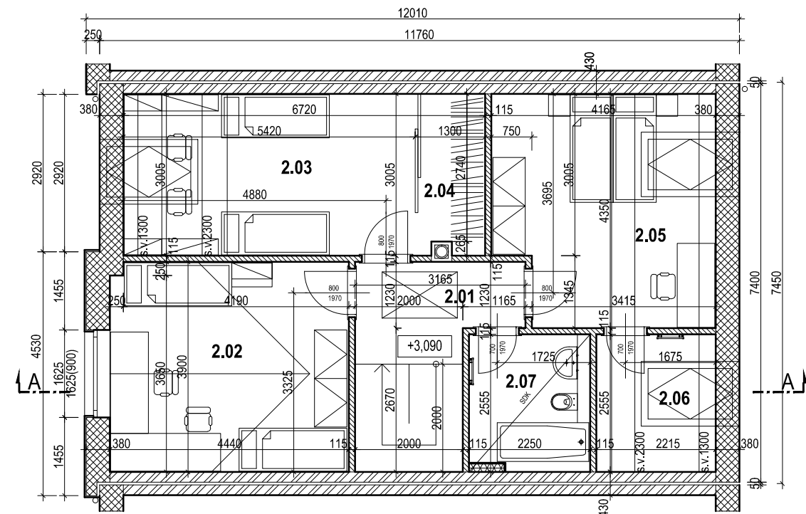
2. NADZEMNÍ PODLAŽÍ
