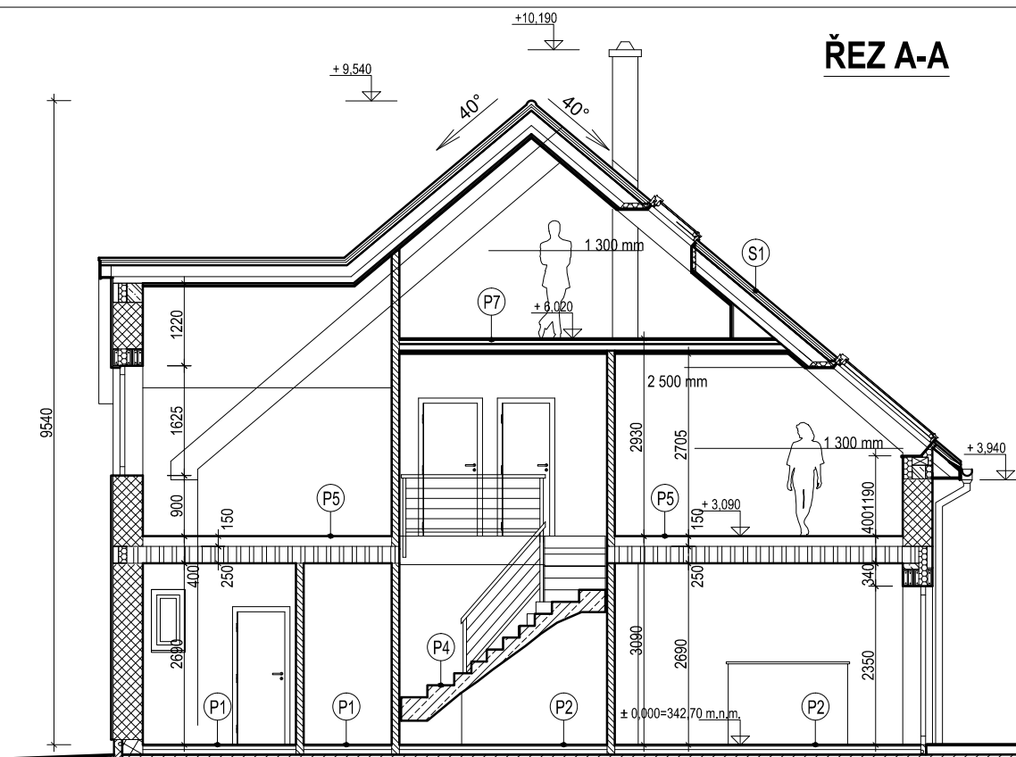
1. NADZEMNÍ PODLAŽÍ
