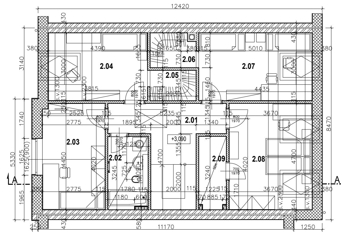
2. NADZEMNÍ PODLAŽÍ
