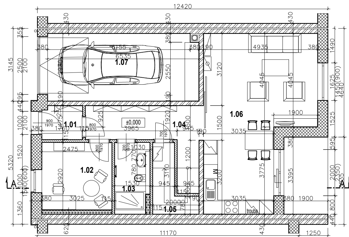
1. NADZEMNÍ PODLAŽÍ
