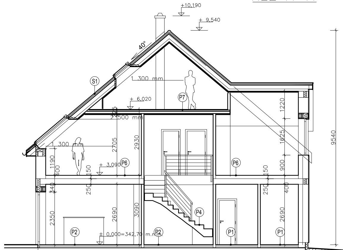
1. NADZEMNÍ PODLAŽÍ
