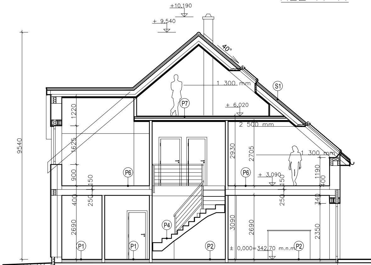
1. NADZEMNÍ PODLAŽÍ
