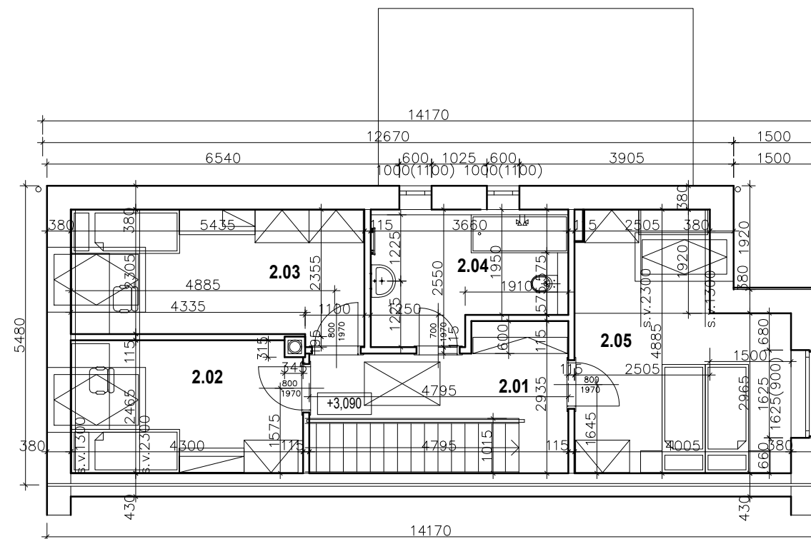
2. NADZEMNÍ PODLAŽÍ
