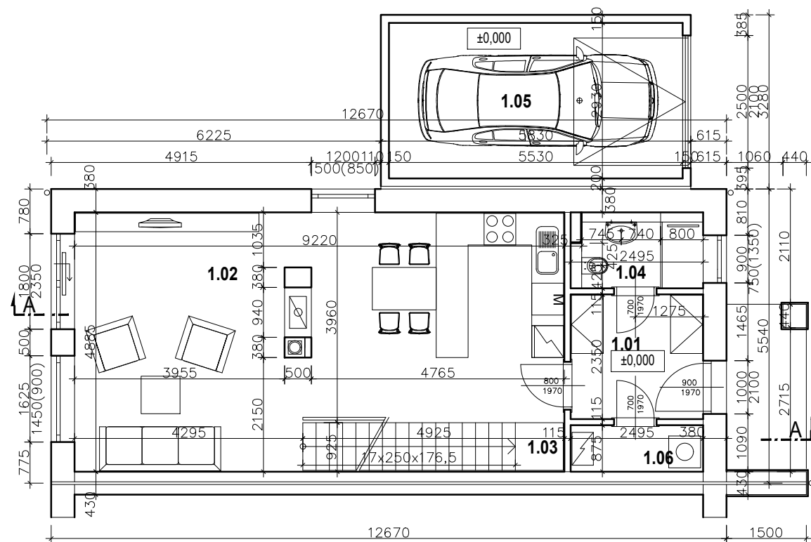
1. NADZEMNÍ PODLAŽÍ
