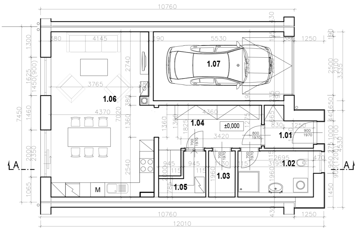
1. NADZEMNÍ PODLAŽÍ
