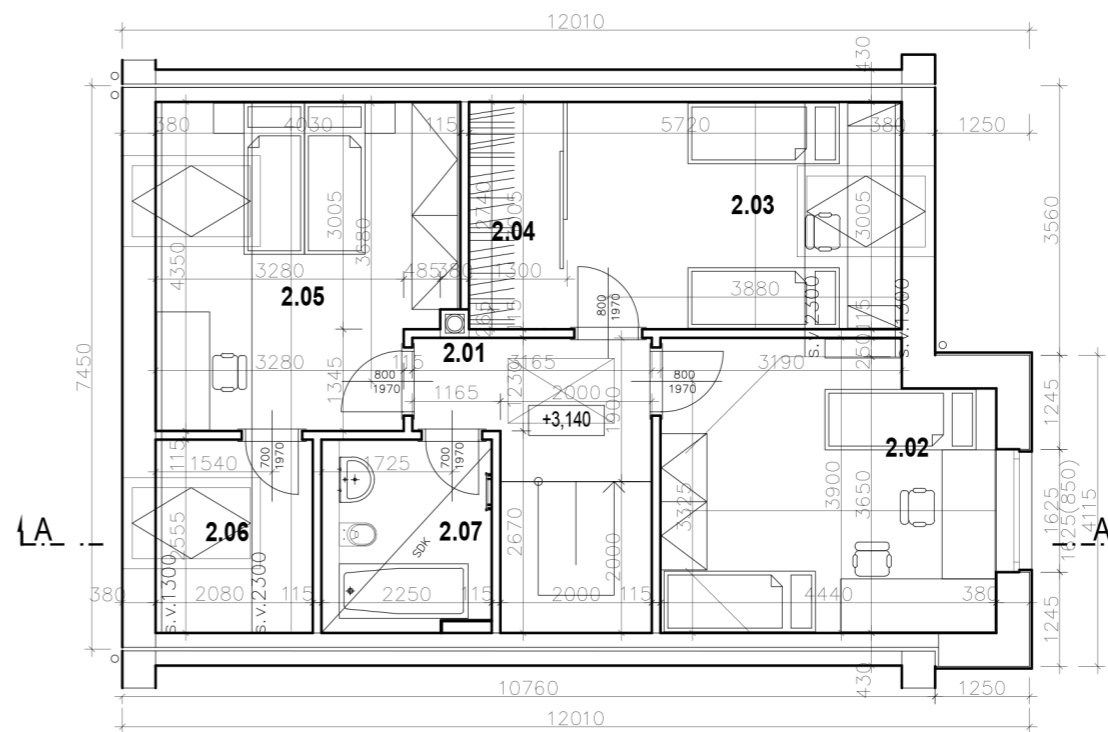
2. NADZEMNÍ PODLAŽÍ
