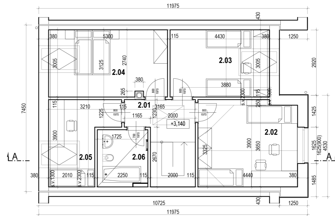
2. NADZEMNÍ PODLAŽÍ
