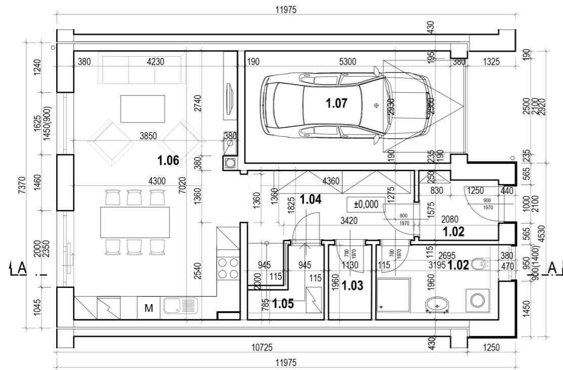
1. NADZEMNÍ PODLAŽÍ
