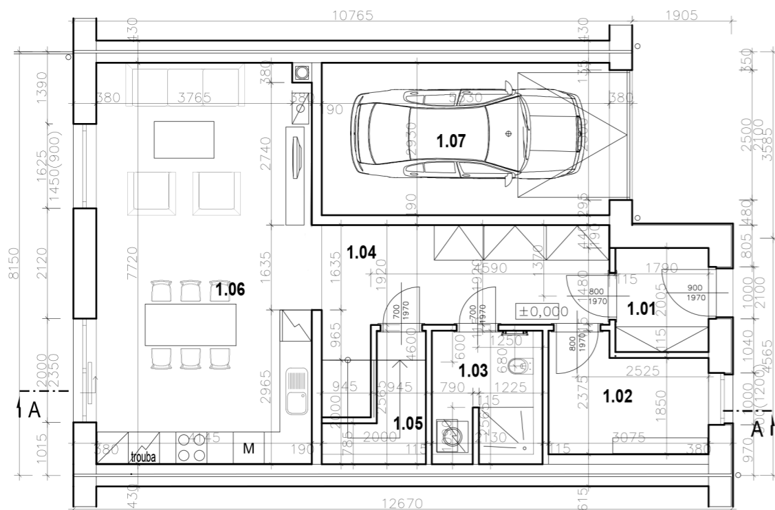
1. NADZEMNÍ PODLAŽÍ
