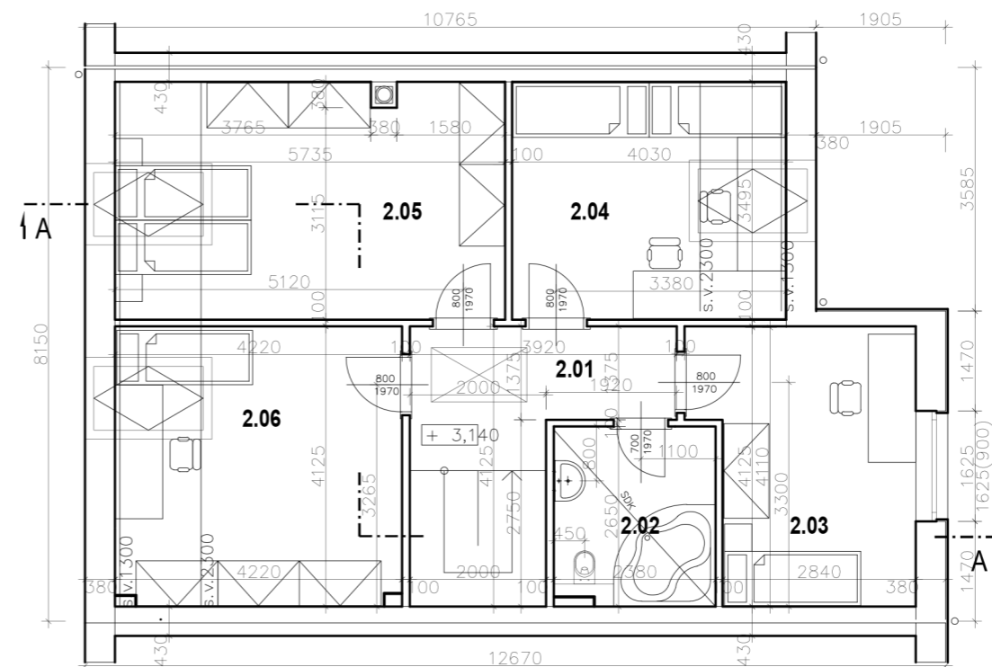
2. NADZEMNÍ PODLAŽÍ
